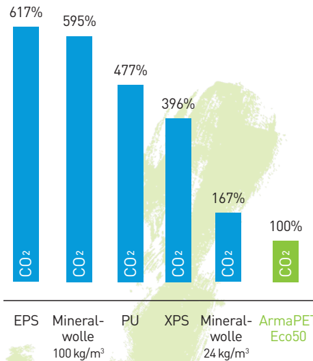
Standard-Dämmstoffe
