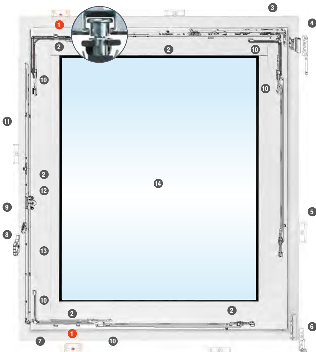
1 + 2 Pilzkopfverriegelung
