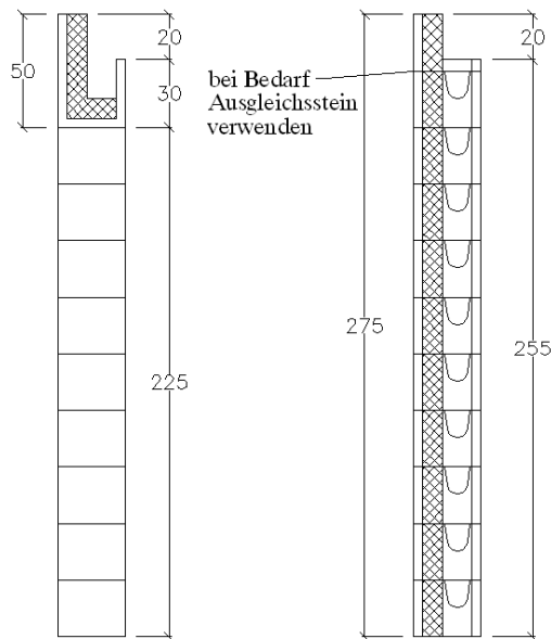
Schnitt 3-3
