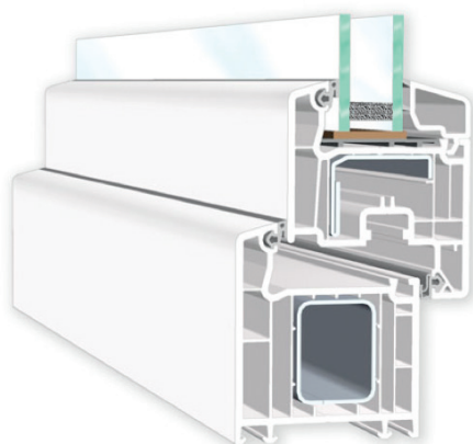
SOFTLINE (Flügel flächenversetzt)
