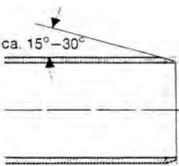
Abb. 53: Einschubende anschrägen
