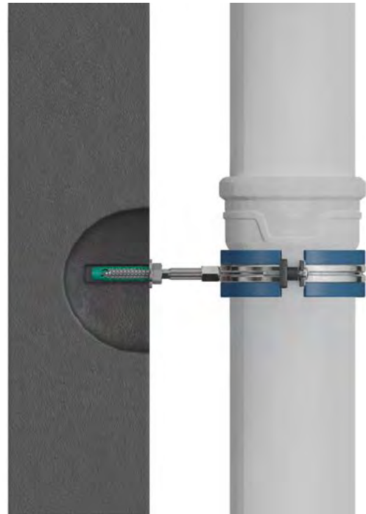
Zusätzliche Fallrohrsicherung mit Hilfe einer Festpunktauflage
