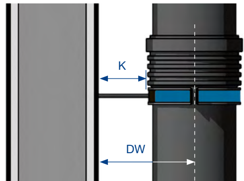
Vertikaler Abstand von der Rohrschelle zum Mauerwerk
