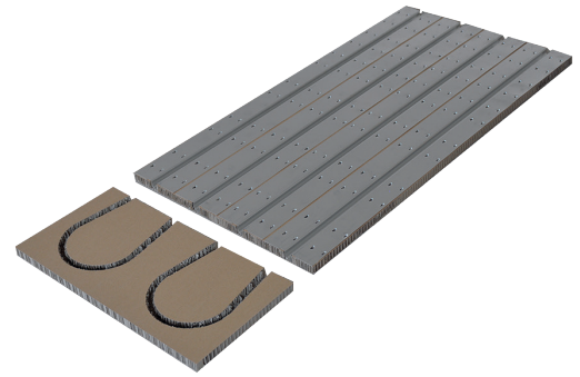
Rohrabstand 125 mm
