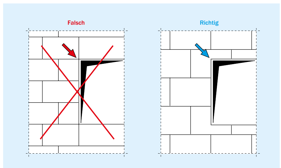
Bild 27 Stoßfugenfreie Verlegung von WDVS-Dämmplatten im Bereich von Wandöffnungssecken
