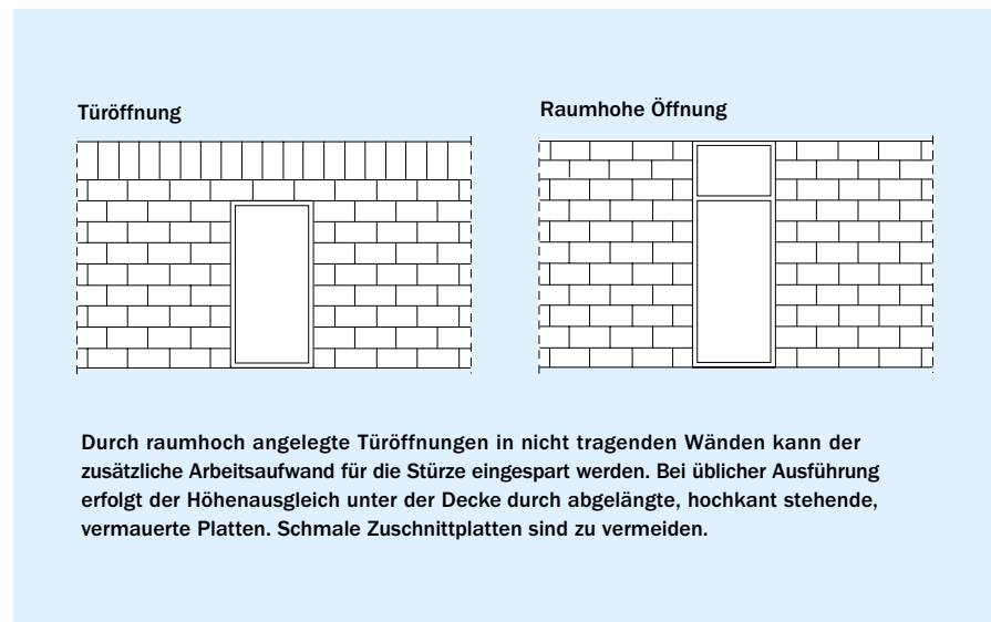
Bild 9 Türöffnungen
