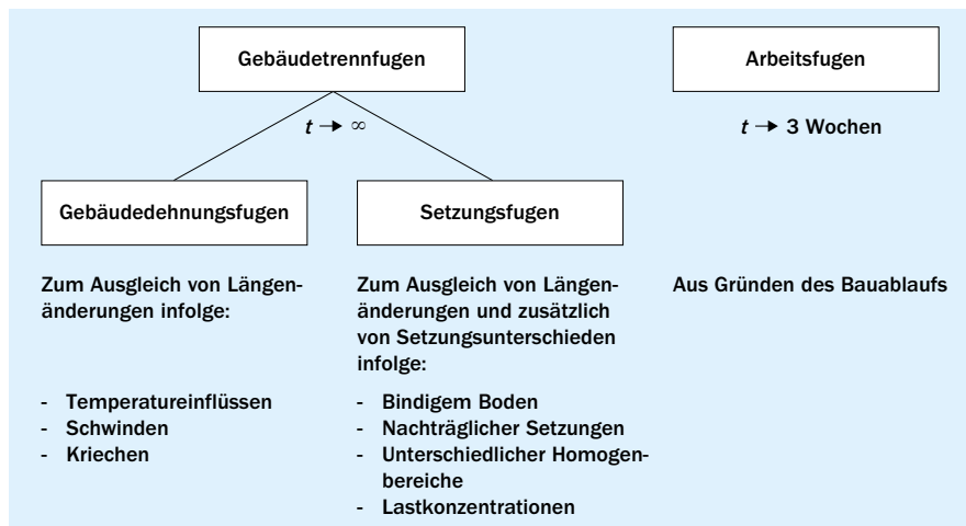
Bild 35 Gebäudegliederung durch Fugen
