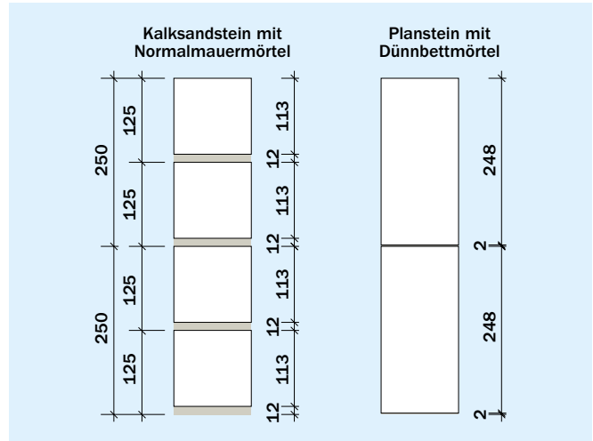
Bild 25 Schichtmaß
