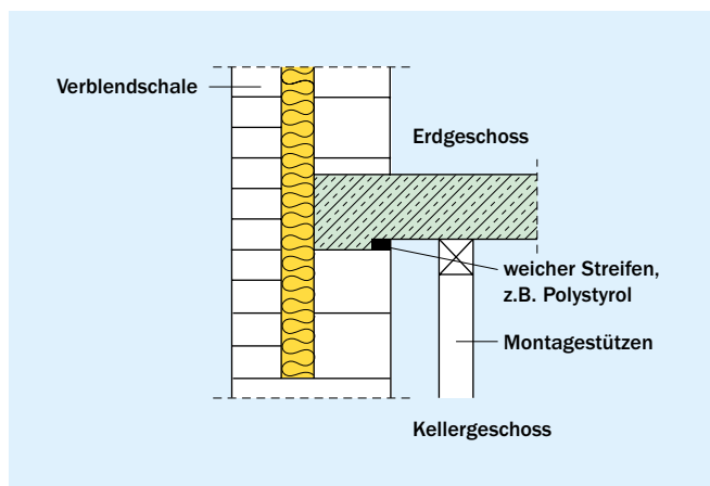
Bild 31 Konstruktive Zentrierung
