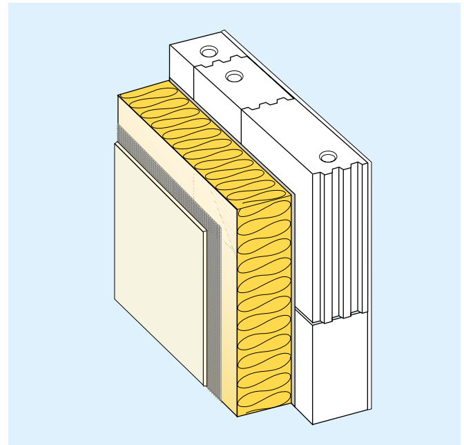
Bild 10 Kalksandstein-Mauerwerk mit Wärmedämm-Verbundsystem (WDVS)
