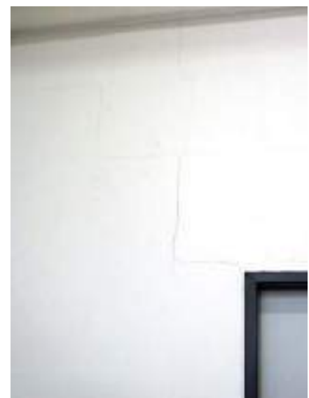
Bild 24 Rissbildung in nicht tragender Trennwand infolge Durchbiegung der unteren Geschossdecke
