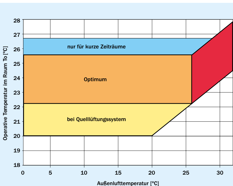
Bild 14 Zulässigkeitsbereich der operativen Temperatur in Abhängigkeit von der Außenlufttemperatur nach DIN 1946-2
