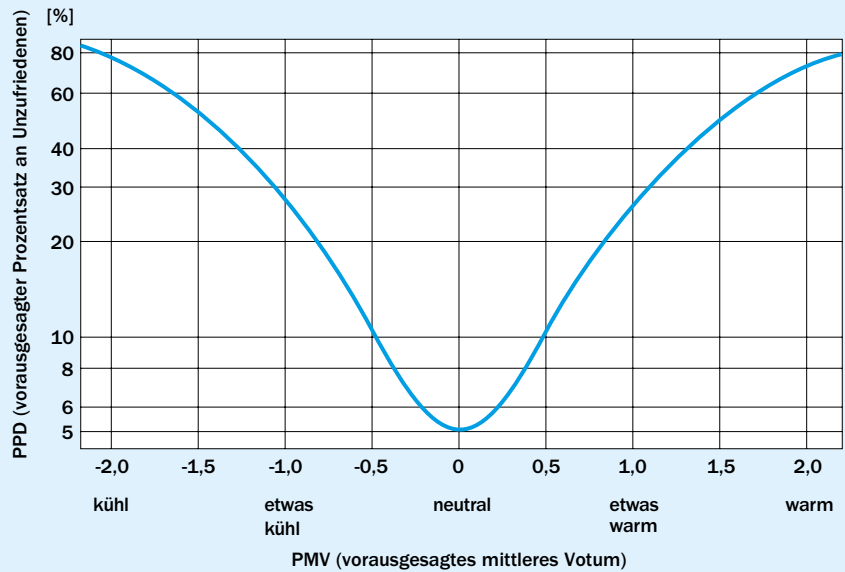
Bild 13 Vorausgesagter Prozentsatz an Unzufriedenen (PPD) in Abhängigkeit vom mittleren Votum PMV
