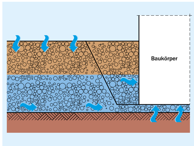
Bild 7 Drückendes Wasser unter der Bodenplatte
