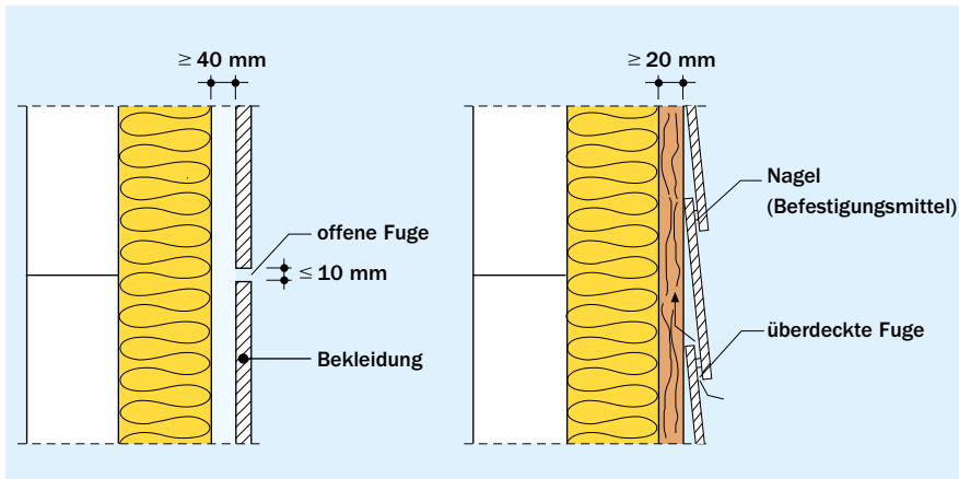
Bild 47 Fugenausbildung bei hinterlüfteten Bekleidungen (aus [35])
