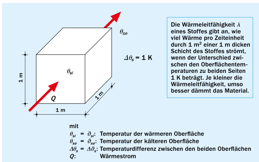
Bild 3 Wärmeleitfähigkeit
