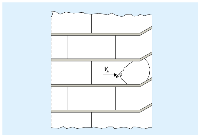
Bild 8 Steinkantenbruch am Mauerwerksrand [9]
