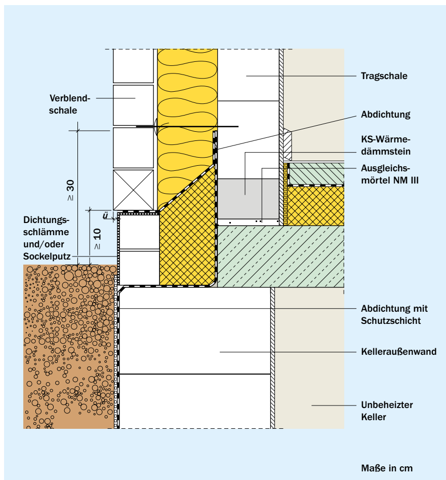
Bild 11 Beispiel für Fußpunktausbildung bei zweischaligem Mauerwerk
