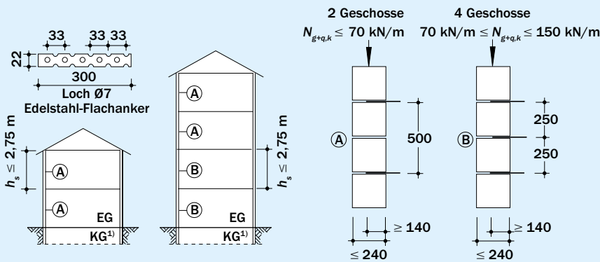
Bild 38 KS-Stumpfstoßtechnik, Regelausführung bei Annahme einer drei- oder vierseitigen Halterung der tragenden Wand (Schichthöhe \leq 25 cm) [3]
