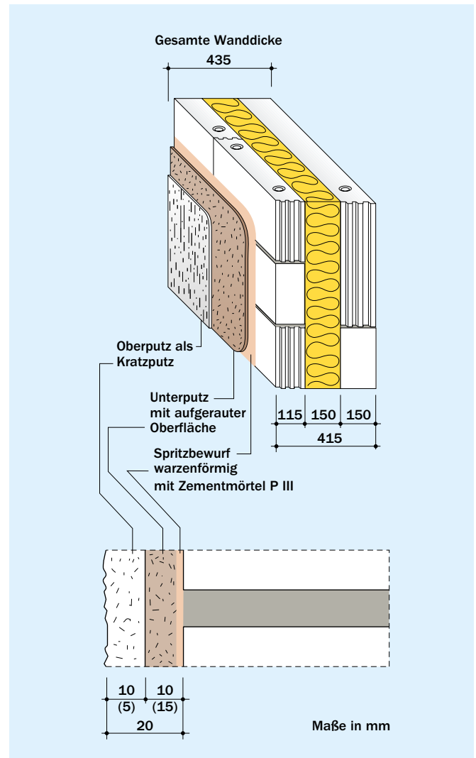
Bild 9 Verputzte Vormauerschale
