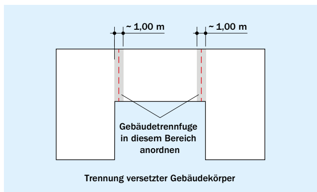
Bild 37 Trennung versetzter Gebäudekörper mit Gebäudetrennfugen
