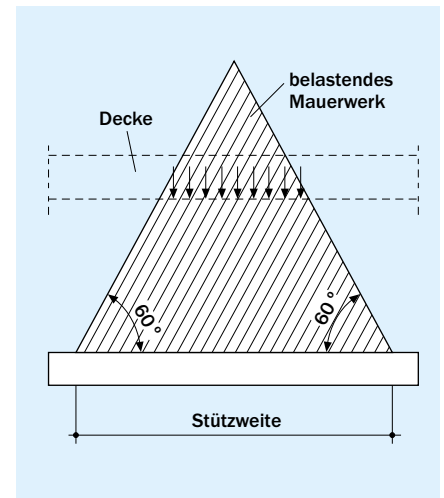
Bild 27 Ermittlung der Belastung von Flachstürzen für l_{0f} \geq 0,4 \cdot h_v
