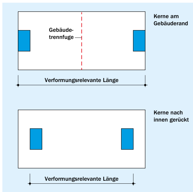
Bild 36 Auswirkung des Gebäudegrundrisses auf die Anordnung von Dehnungsfugen
