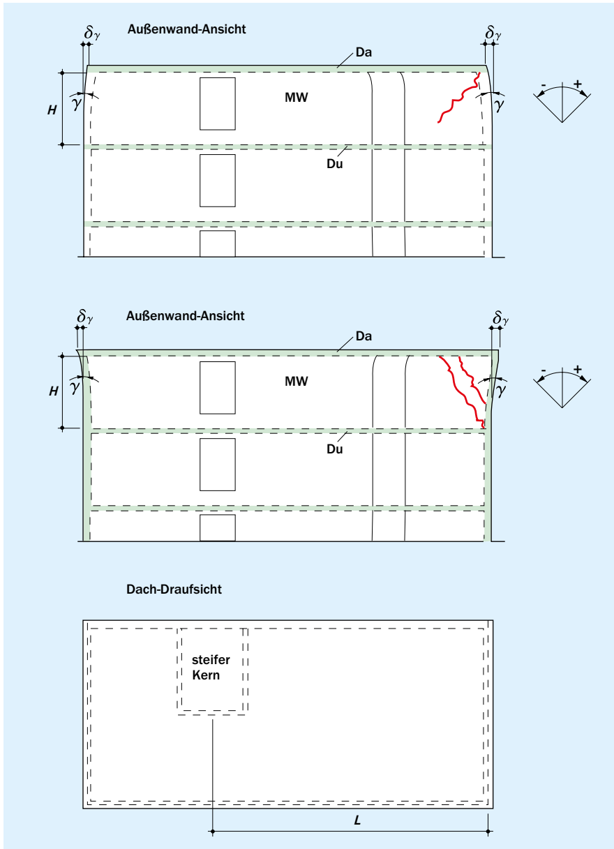
Bild 14 Verformungsfall H3: Verformung der Dachdecke gegenüber der Wand; Da = Dachdecke, Du = Decke unter Da, MW = Mauerwerkswand
